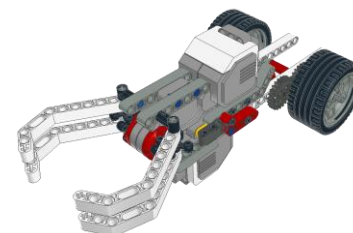
オリジナル教材（ギアを学ぶ カブト・クワガタロボ）
